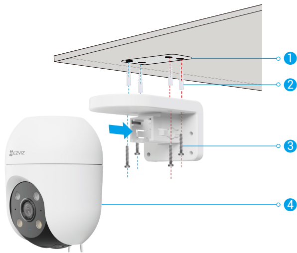
그림 1 천장 장착
