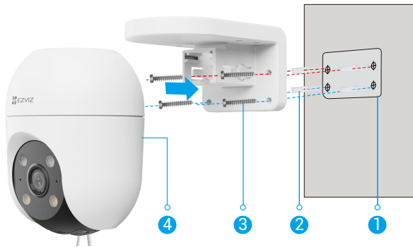
그림 2 벽 장착
